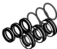
P9.003.009 GUARNIZIONE PISTONE ø25 POMPA GM-1 - KIT PLUNGER SEALS
